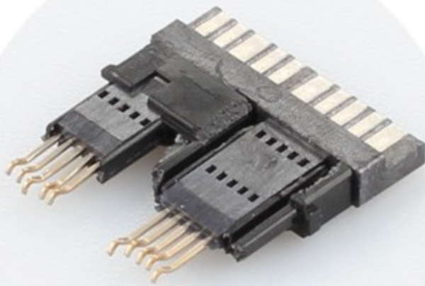
内部结构
